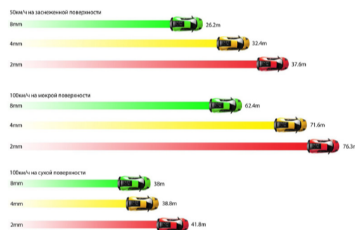
Длина тормозного пути на разном покрытии в зависимости от глубины протектора
